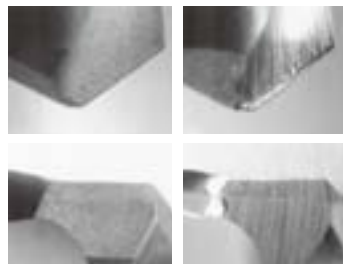
ダイヤコーティングドリル Diamond Coated Drill
