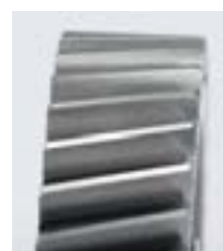
シェービング後加工面 After Shaving
