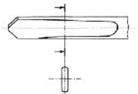
(a) フラットドリル
