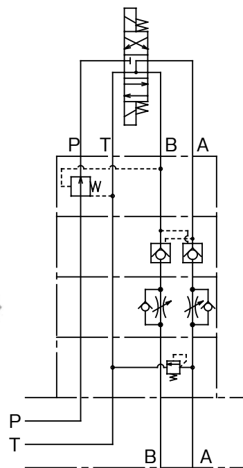
集積化回路図
