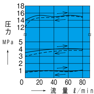
OCQ-G03-A1*-J50 ー圧力上昇 ー圧力下降
