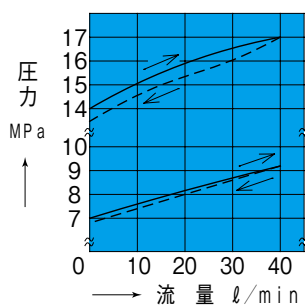
OCQ-G01-A1*-20 ー圧力上昇 ー圧力下降
