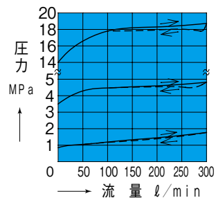
OQH-G04-A1*-10 ー圧力上昇 ー圧力下降
