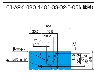
バルブ取付面寸法
