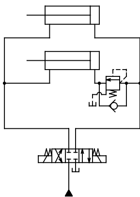
回路例1 タイプ2を使用の場合
