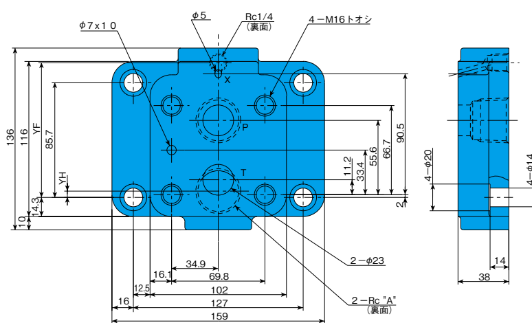
サブプレート MRI-06*-10 (最高使用圧力25MPa)
