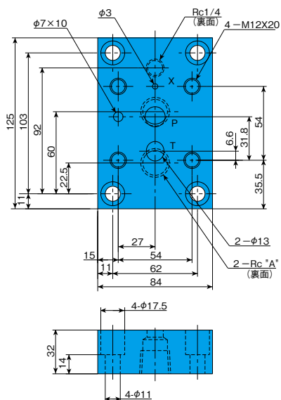
サブプレート MRI-03*-10 (最高使用圧力25MPa)
