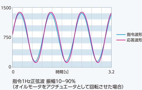
速度正弦波応答
