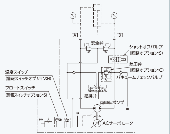
油圧回路図(UPS-0A、1A、2A)
