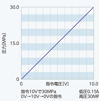
圧力指令電圧-圧力特性(0-100%)
