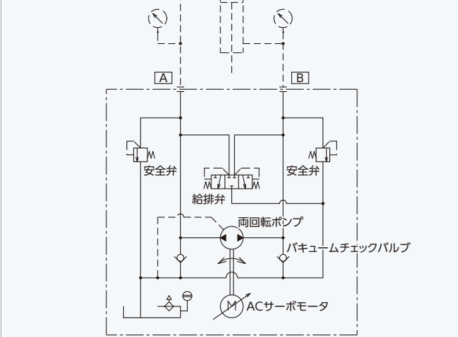
油圧回路図(UPS-00A)
