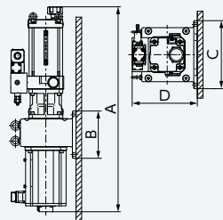
垂直取付
