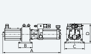
水平取付
