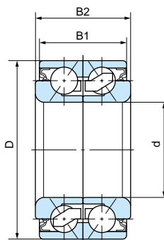
形式 B (両接触シール形)
