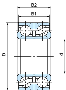
形式 A (開放形)
